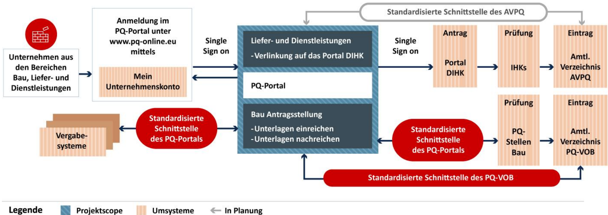
Abbildung 2: Funktionsübersicht des Online-Dienstes Präqualifizierungsservice
