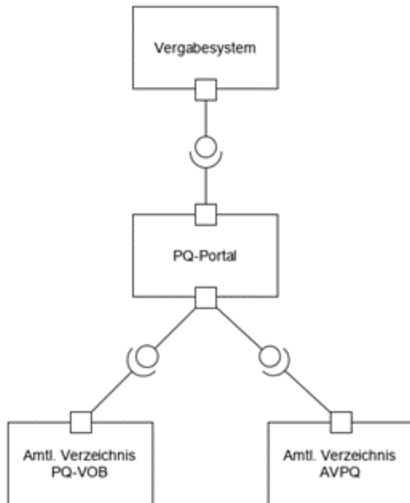
Abbildung 10: Schnittstellen-Architektur schematisch
